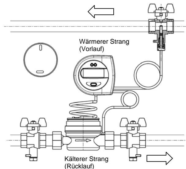
Abb. 1: Einbau PolluCom E/S im Rücklauf einer Heizungsanlage, Vorlauftemperaturfühlereinbau im Kugelhahn
