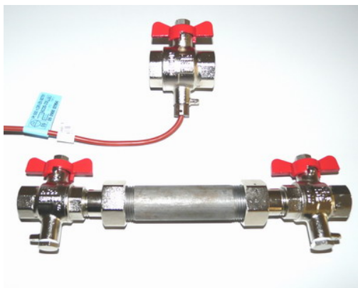
Abb. 2 MID Erstausrüster-Set
